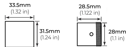
END CAP
