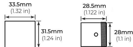
END CAP
